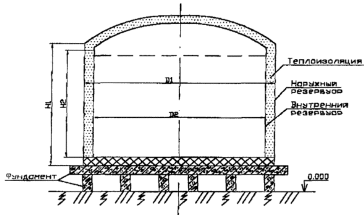
Эскиз двустенного ИР с подвесной внутренней крышей
