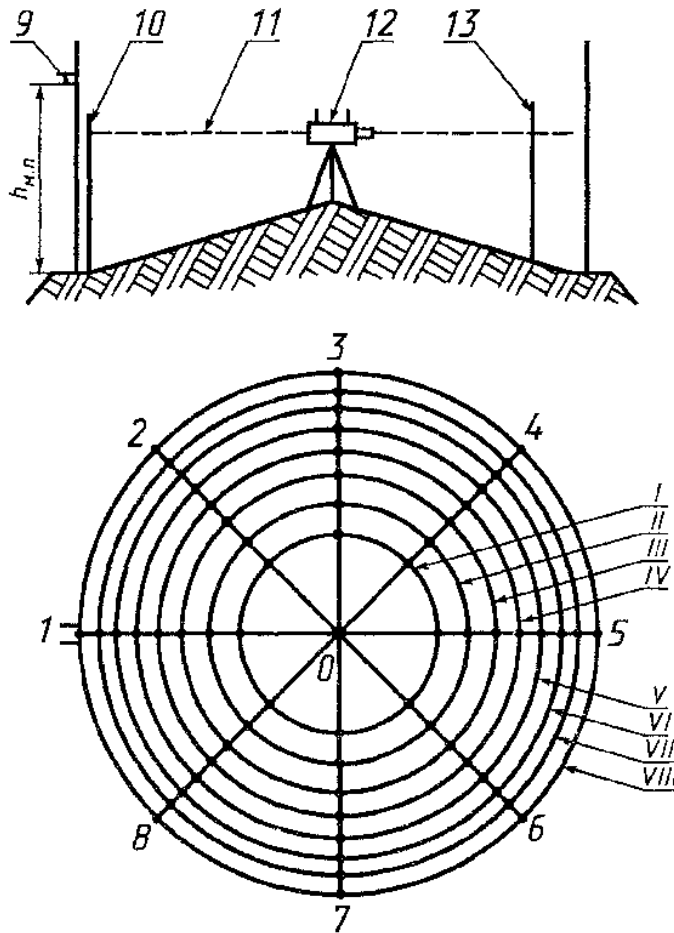
Рисунок А.13 - Схема расположения поясов резервуара
