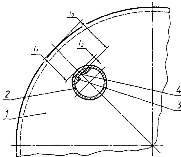
Рисунок А.15 - Нивелирование дна резервуара при наличии центральной трубы
