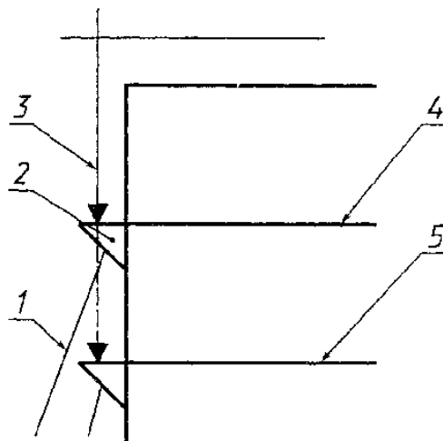
Рисунок А.11 - Схема определения степени наклона резервуара с применением отвеса
